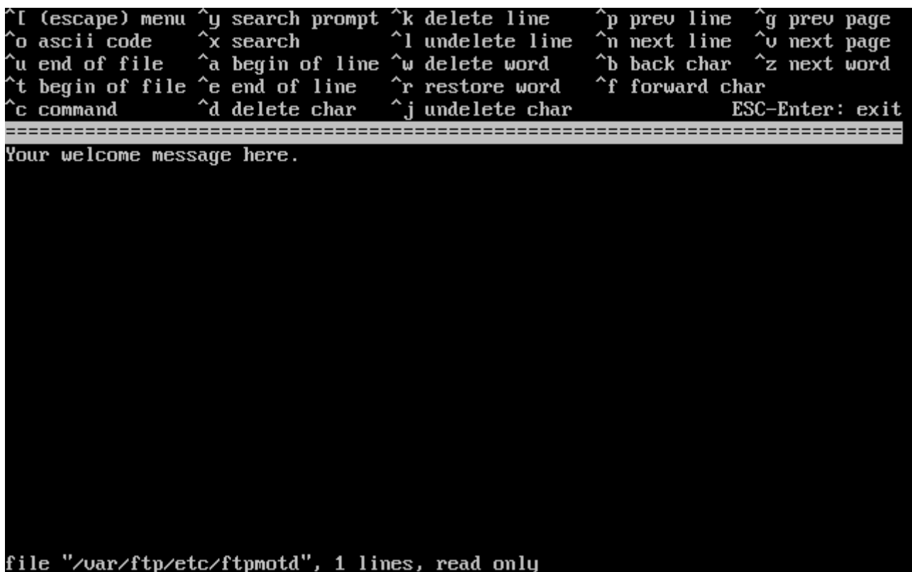
Рисунок 31. Редактирование FTP Welcome Message
