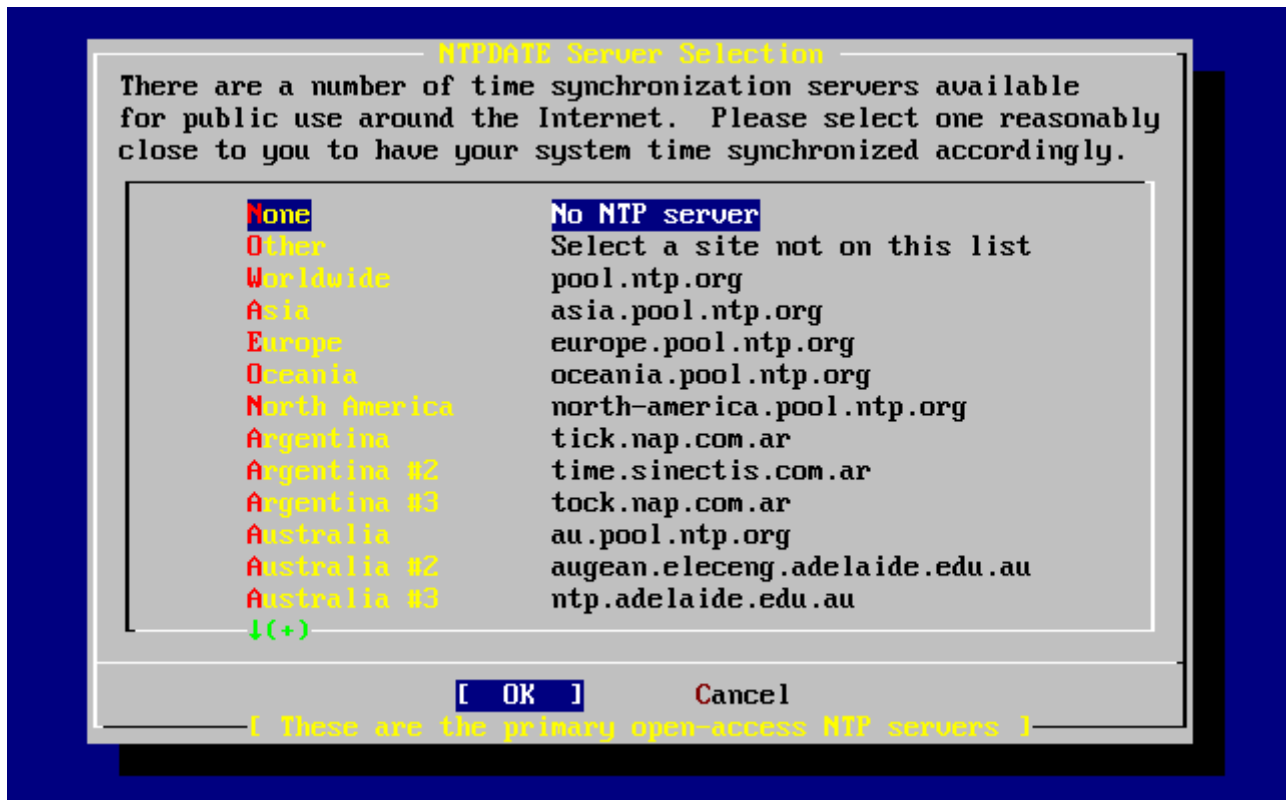
Рисунок 56. Настройка Ntpdate
